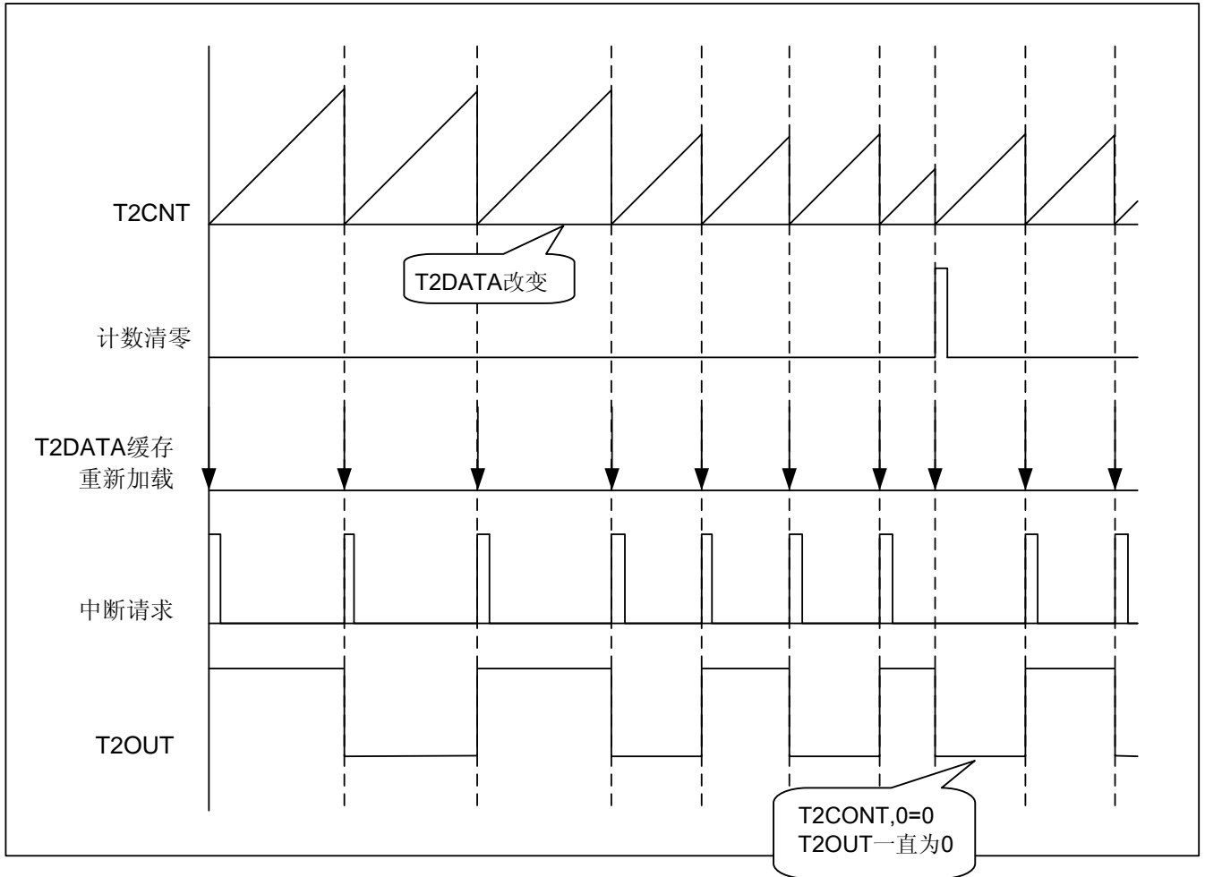
TMR2 时序图
